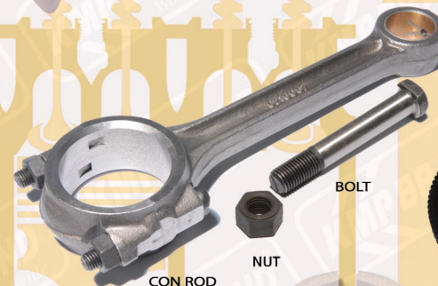
CON ROD
